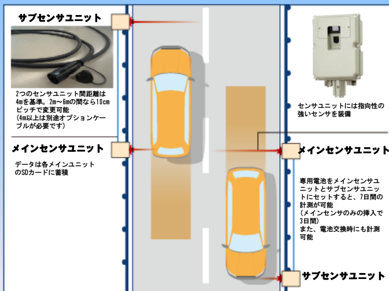
片側1車線2車線計測例
